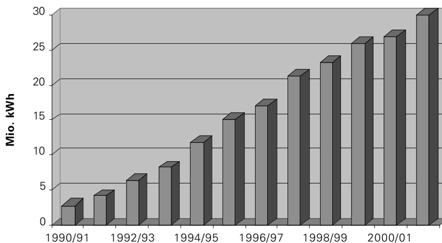
Gasverbrauch
