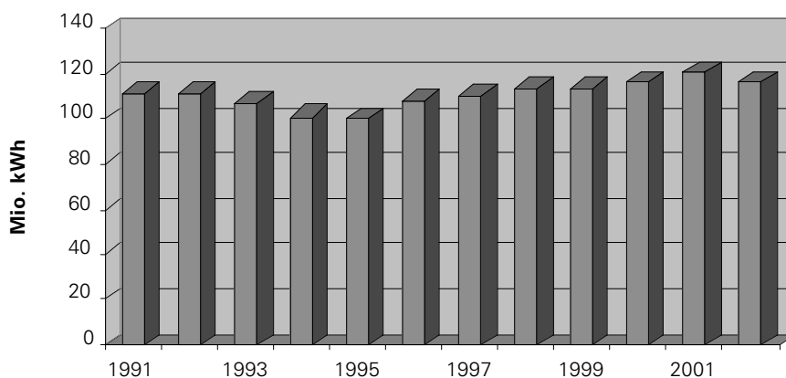
Stromverbrauch
