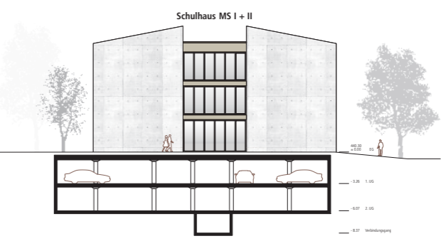
Fassadenansicht Nord
