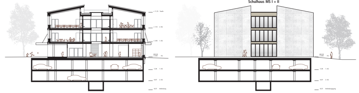
Schnitt F-F
