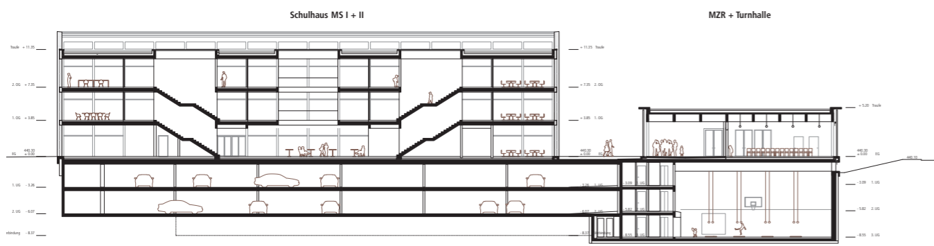
Schnitt D-D
